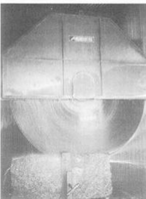
"Granitex": sterowana przez komputer pila firmy "ARBES" o średnicy 2700 mm do przecinania bloków na płyty
